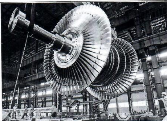
上图为汽轮机装置外观
